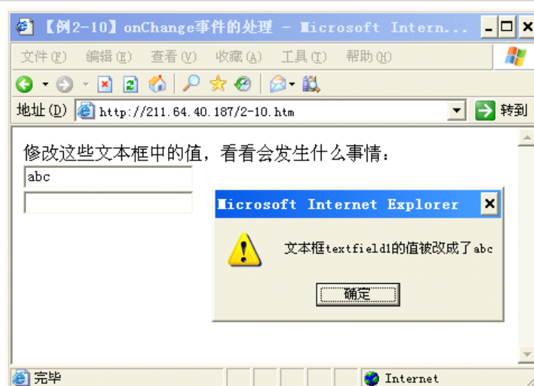
onChange 事件
