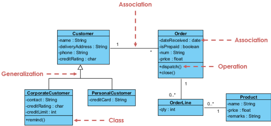
图 1：类图示例（图片来自 Visual Paradigm）
