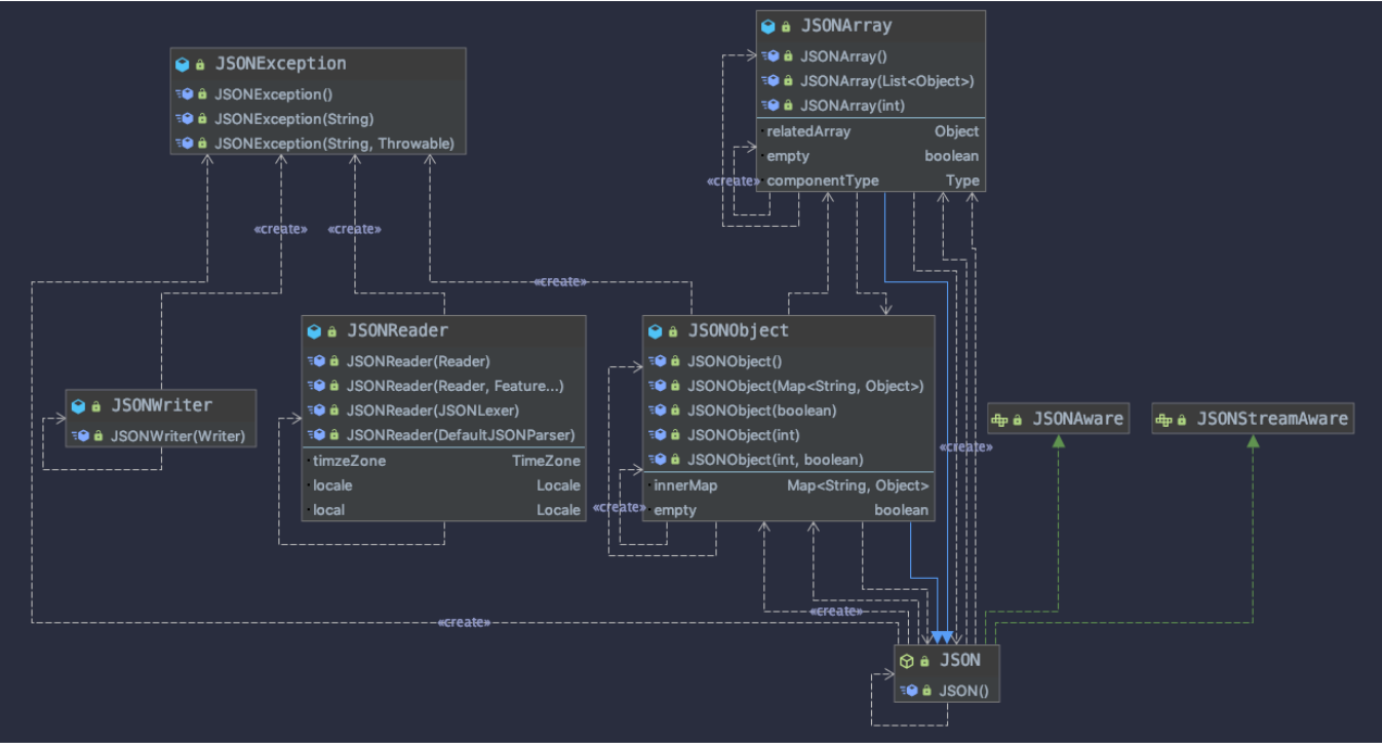
图 13 : fastjson 核心类的类图
