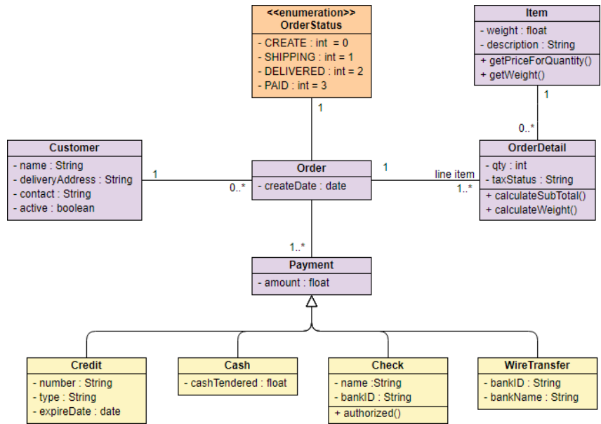
图 1：类图示例（图片来自 Visual Paradigm）
